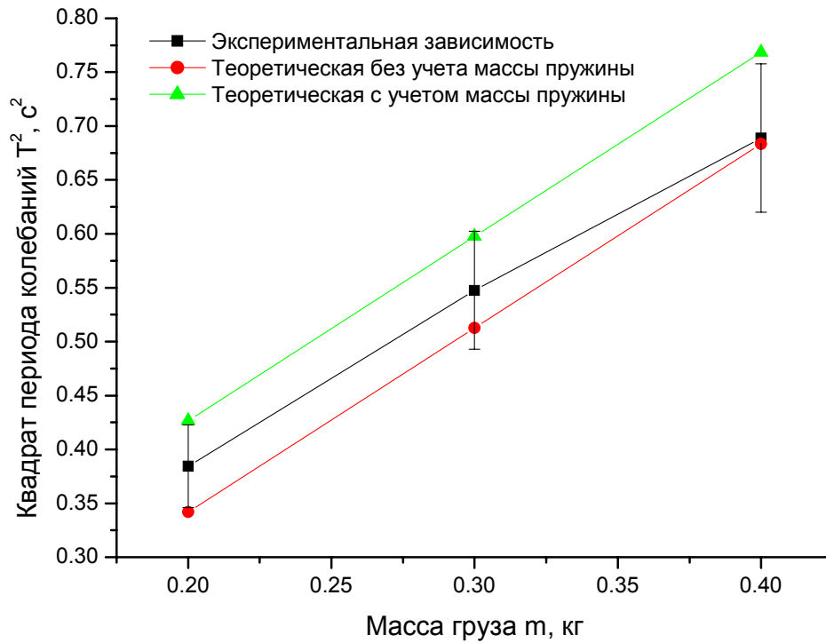
Зависимость квадрата периода колебаний от массы груза для пружины m = 149 г
