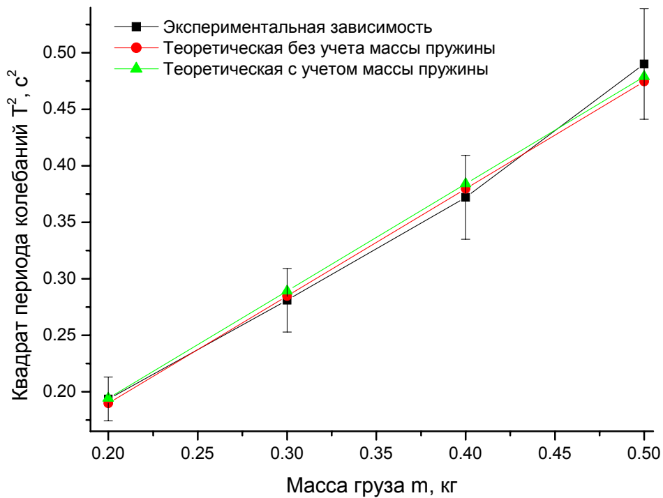
Зависимость квадрата периода колебаний от массы груза для пружины m = 14 г
